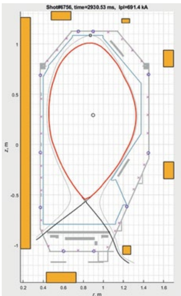
Восстановленная форма поперечного сечения плазменного шнура КТМ
