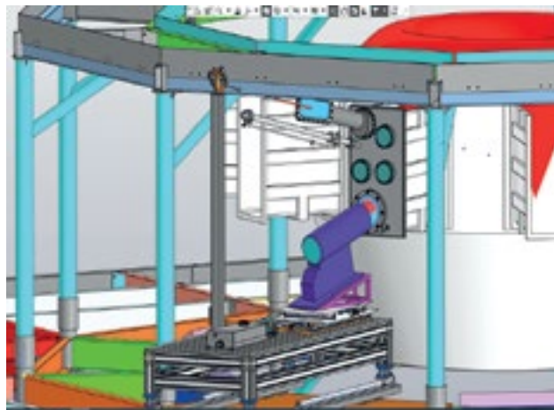
Модель размещения основного оборудования диагностики томсоновского рассеяния на токамаке КТМ
