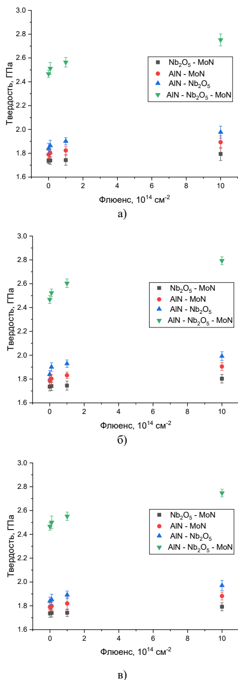
Рисунок 1. Результаты оценки механических свойств: а) облучение ионами N^+ ; б) облучение ионами C^+ ; в) облучение ионами O^+
