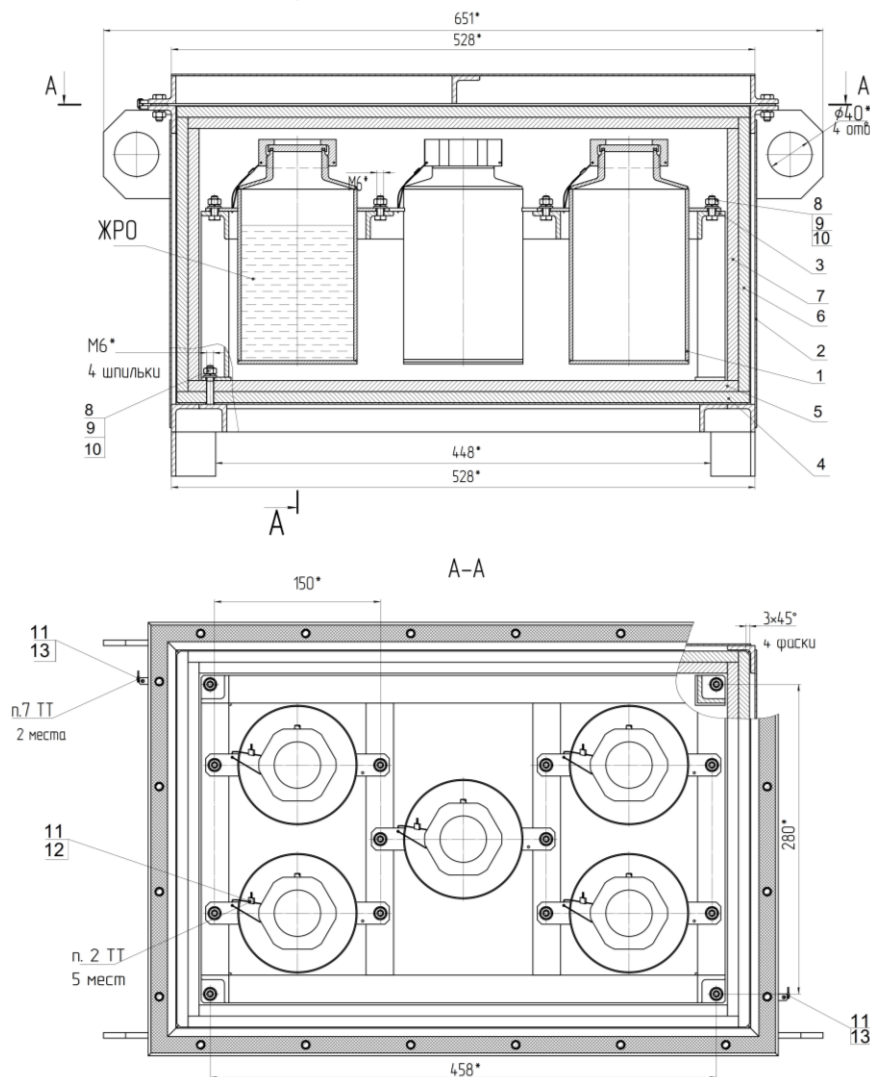
1 – емкость; 2 – контейнер; 3 – каркас; 4, 5 – плита нижняя; 6, 7 – плита боковая; 8 – гайка; 9 – шайба; 10 – болт; 11 – прокладка; 12, 13 – проволока
