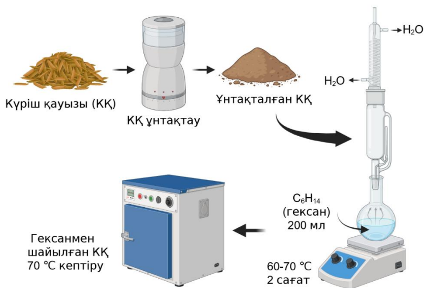
Сурет 1. БМ-ды ұнтақтау және гексанмен шаяу процестер
