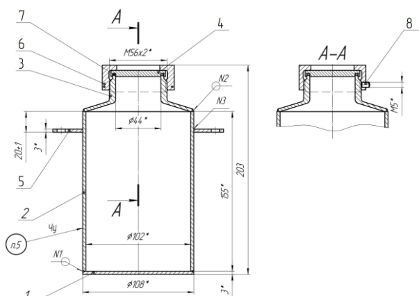
1 – днище; 2 – обечайка; 3 – горловина; 4 – крышка; 5 – кронштейн; 6 – гайка; 7 – прокладка; 8 – винт
