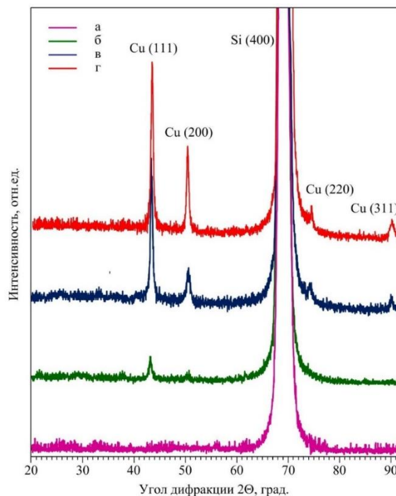
Рисунок 2. Дифрактограммы образцов ПК (а) до и после их выдержки в спиртовом растворе для химического контактно-обменного осаждения меди в течение 1 (б), 3 (в) и 5 (г) минут
