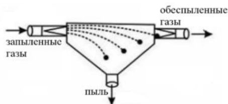
Рисунок 2. Гравитационное осаждение
