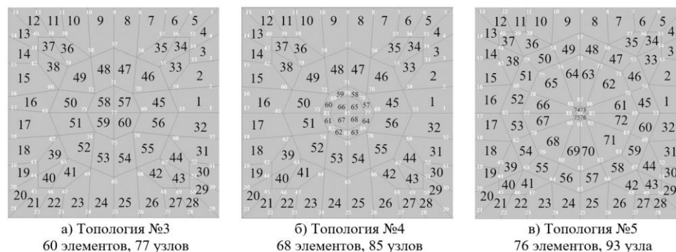
Рисунок 8. Топологии графитовых блоков отражателя
