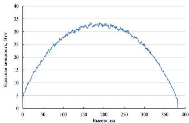
Рисунок 10. Высотное распределение средней удельной мощности в твэлах, размещенных в составе модели реактора APR-1400 (слева) и ОУ в реакторе ИГР (справа)
