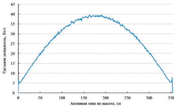
Рисунок 9. Высотное распределение средней удельной мощности в твэлах, размещенных в составе модели реактора ВВЭР-1000 (слева) и ОУ в реакторе ИГР (справа)
