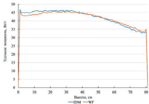
Рисунок 11. Высотное распределение средней удельной мощности в твэлах, размещенных в составе модели реактора HPR-1000 (слева) и ОУ в реакторе ИГР (справа)
