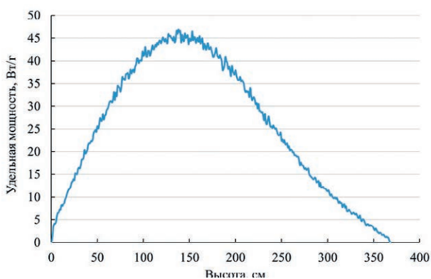
Рисунок 11. Высотное распределение средней удельной мощности в твэлах, размещенных в составе модели реактора HPR-1000 (слева) и ОУ в реакторе ИГР (справа)
