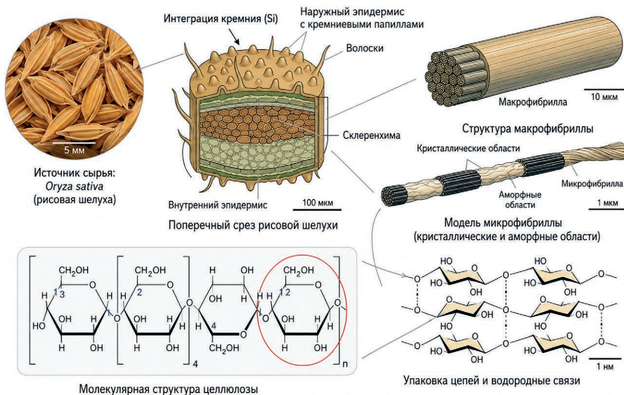
Рисунок 1. Иерархическая структура целлюлозы на примере рисовой шелухи ( Oryza sativa ): источник, поперечный срез с кремнезёмными папиллами, макро- и микрофибриллы, молекулярная структура и водородные связи [8, 9, 24, 42]
