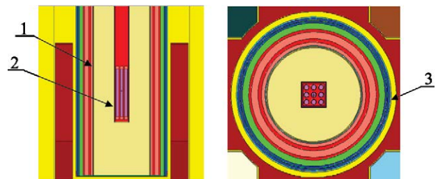
Рисунок 2. поперечное сечение расчетной модели тепловыделяющей сборки, размещенной в реакторе ИГР 1 – ловушка, 2 – ТВС, 3 – НА-228
