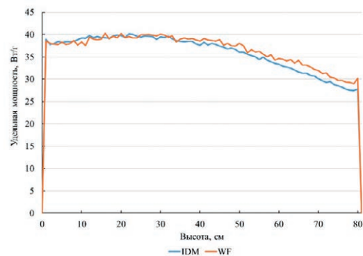
Рисунок 9. Высотное распределение средней удельной мощности в твэлах, размещенных в составе модели реактора ВВЭР-1000 (слева) и ОУ в реакторе ИГР (справа)
