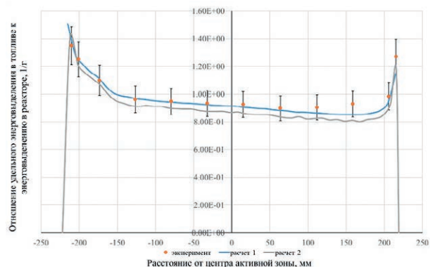
Рисунок 9. Отношение удельного энерговыделения в ТВЭлах модели объекта испытаний с ТВССК 3 ряду
