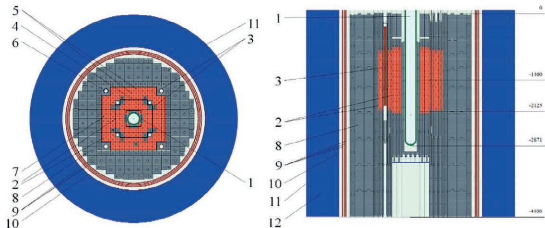
1 – центральный экспериментальный канал (ЦЭК); 2 – активная зона (подвижная и неподвижная части графитовой кладки); 3 – каналы управляющих стержней; 4 – канал физических измерений; 5 – канал термопары; 6 – боковой экспериментальный канал (БЭК); 7 – канал источника нейтронов; 8 – отражатель; 9 – боковая защита (трехслойная оболочка); 10 – кожух реактора; 11 – водяной бак; 12 – полость охлаждающей воды; 13 – ионизационные камеры (ИК); 14 – канал счетчика нейтронов; 15 – биологическая защита; 16 – верхняя защита
