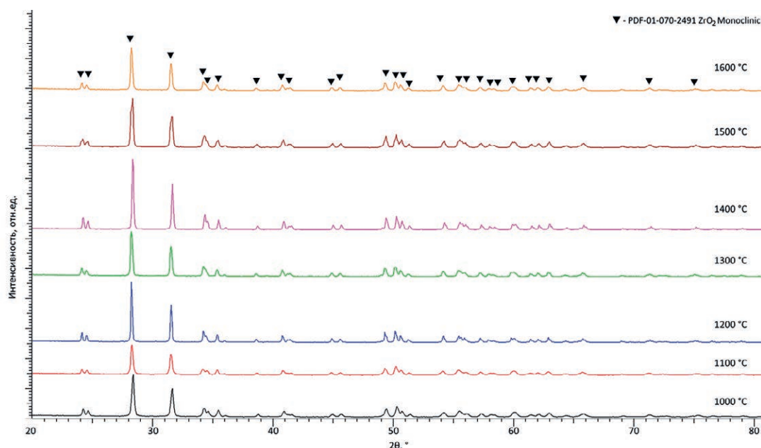
Рисунок 2. Результаты рентгеноструктурного анализа исследуемых ZrO_2 керамик в зависимости от температуры отжига
